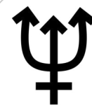
Neptun
