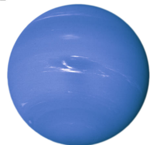
Neptun
