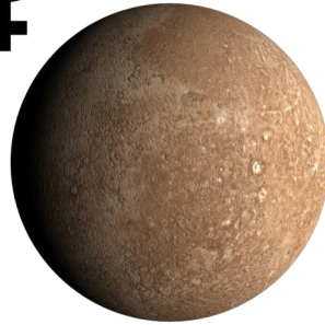
Merkur
