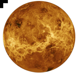
Venuše
